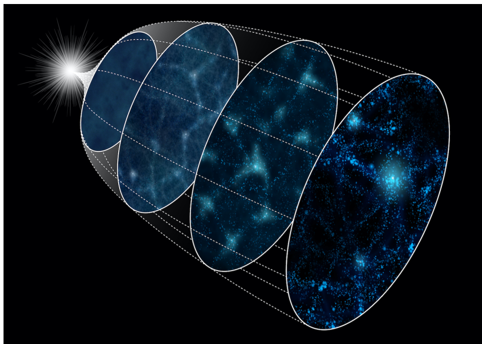
図1：宇宙の大規模構造と再構築法のイメージ図。再構築法は、右前から左奥への移り変わるように、現在の大規模構造の時間をもとに、初期の密度ゆらぎの分布に近づく作用をもつ。（クレジット：統計数理研究所）
