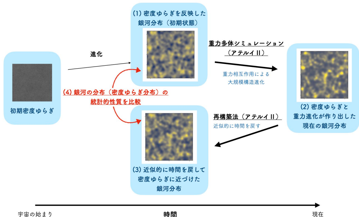
図 2: 本研究の解説図. (1)初期の密度揺らぎが進化したと考え、密度ゆらぎの影響を反映した銀河分布を用意し、それを初期状態として重力多体シミュレーションを行う。(2)密度ゆらぎと、重力相互作用の効果을併せ持った、大規模構造のシミュレーションデータができる。(3)(2)でできた大規模構造のデータに再構築法を適用し、時間を戻すことで、初期の密度ゆらぎの影響を反映した銀河分布に近いものを作り出す。(4)初期状態とした銀河分布と、再構築法で得られた銀河分布を比較し、大変良く似た統計的性質が得られることがわかった。(クレジット: 白崎正人, 国立天文台)
